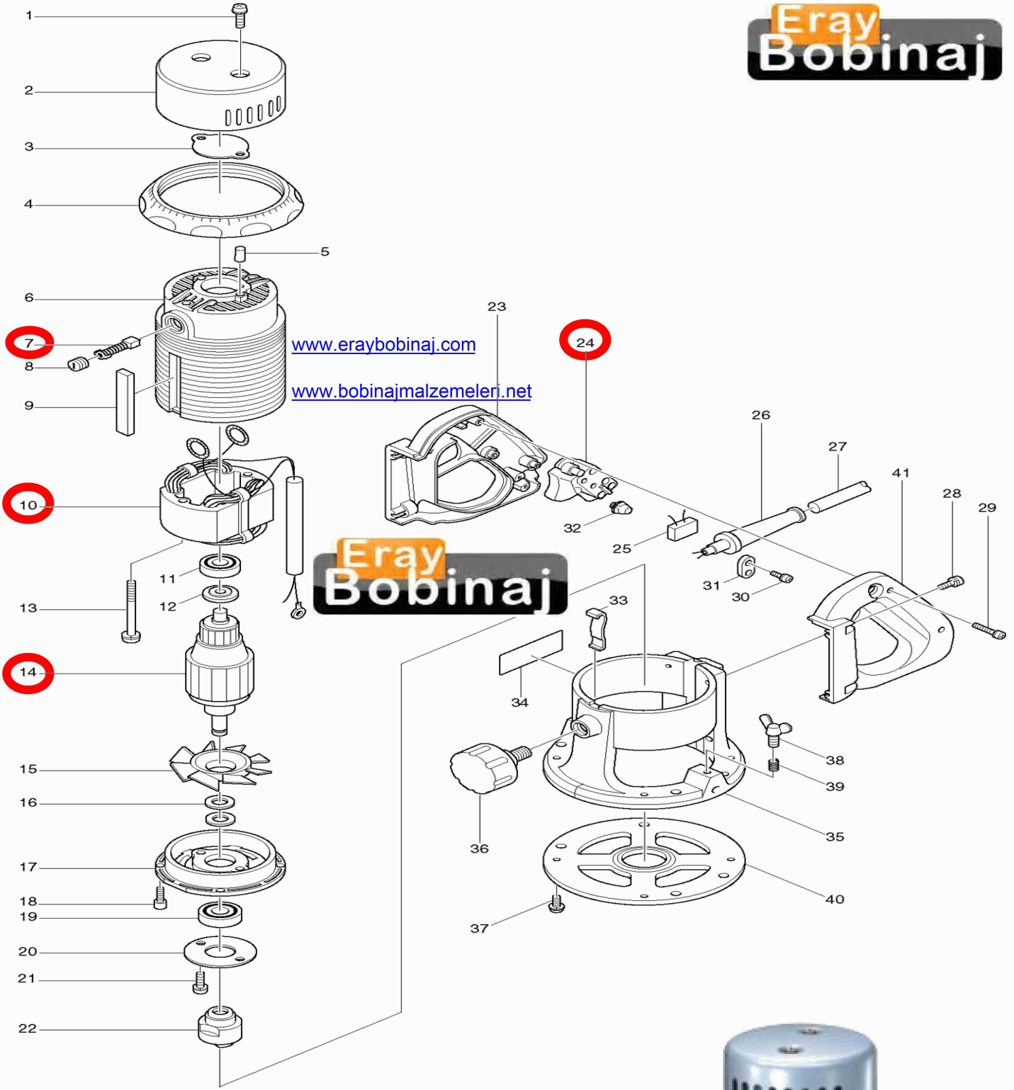
MAKİTA 3601 B FREZE YAN SANAYİ YEDEK PARÇALARI www.eraybobinaj.com
